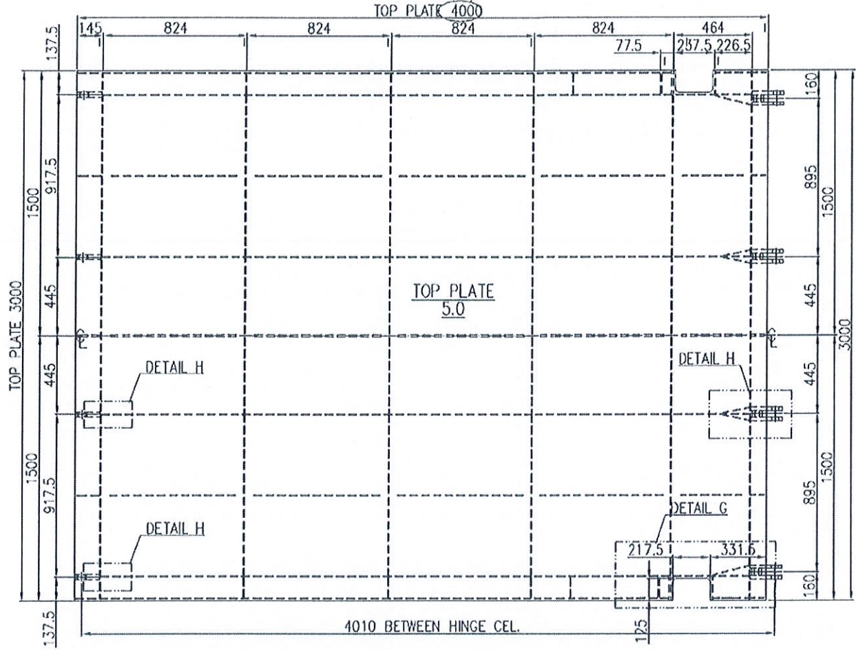
Alüminyum Rampa Konstrüksiyon Resmi
