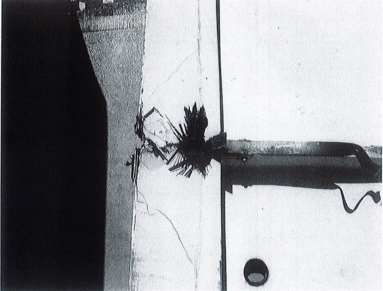
Hasarlı Flap Altı
