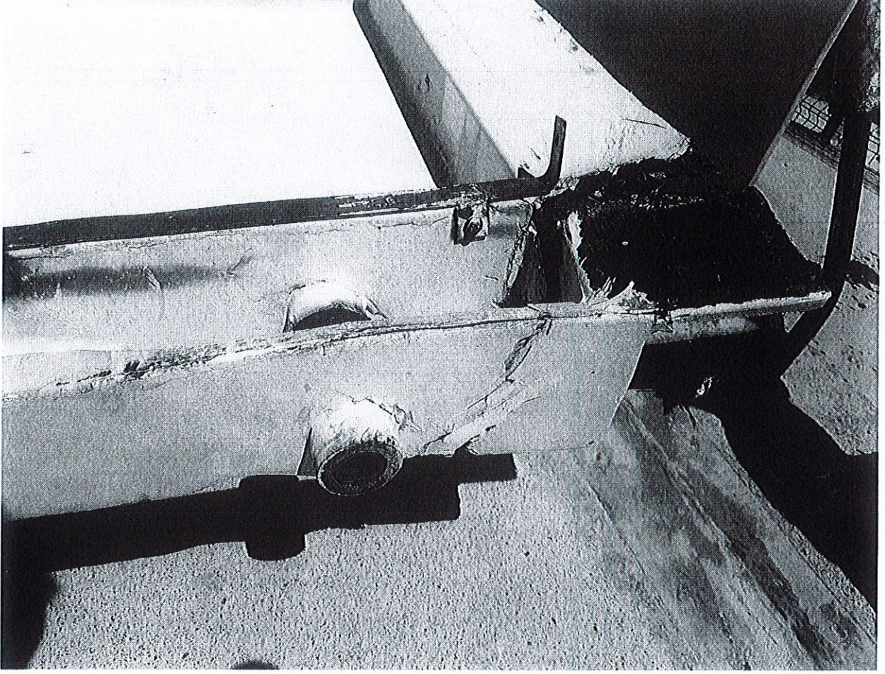
Hasarlı Kompozit Flap Kopan Mentşe Kaynaklı Ayrılma
