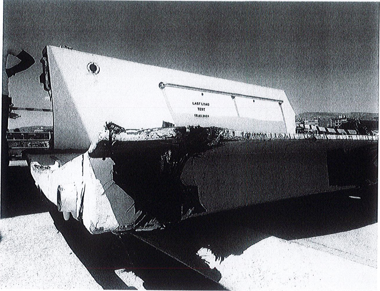
Hasarlı Flap Kopan Menteşe Tarafı
