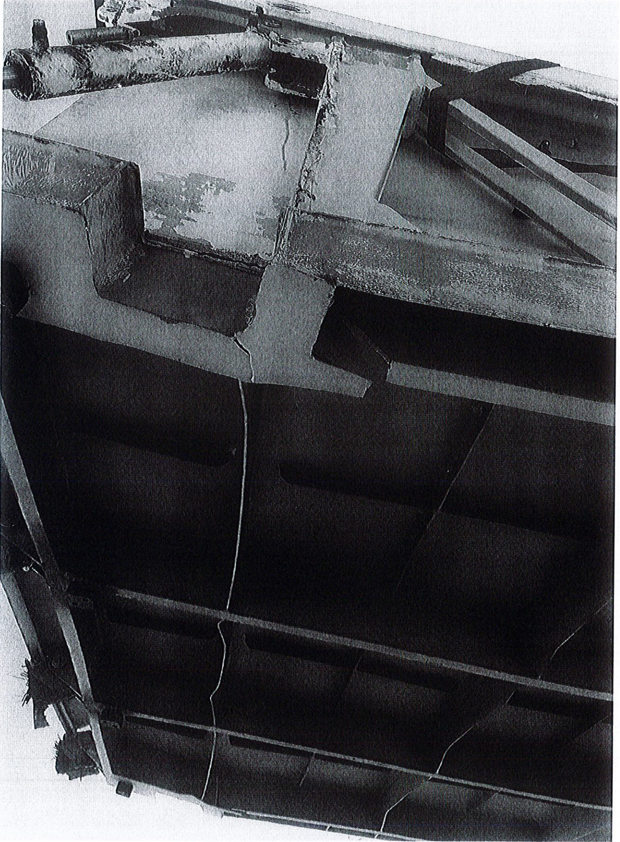
Hasarlı Rampa Alttan Görünüm
