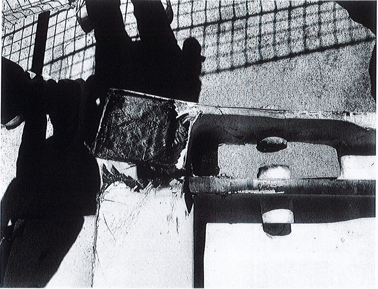
Hasarlı Kompozit Flap Hidrolik Piston Bağlantı Pim Yatağı
