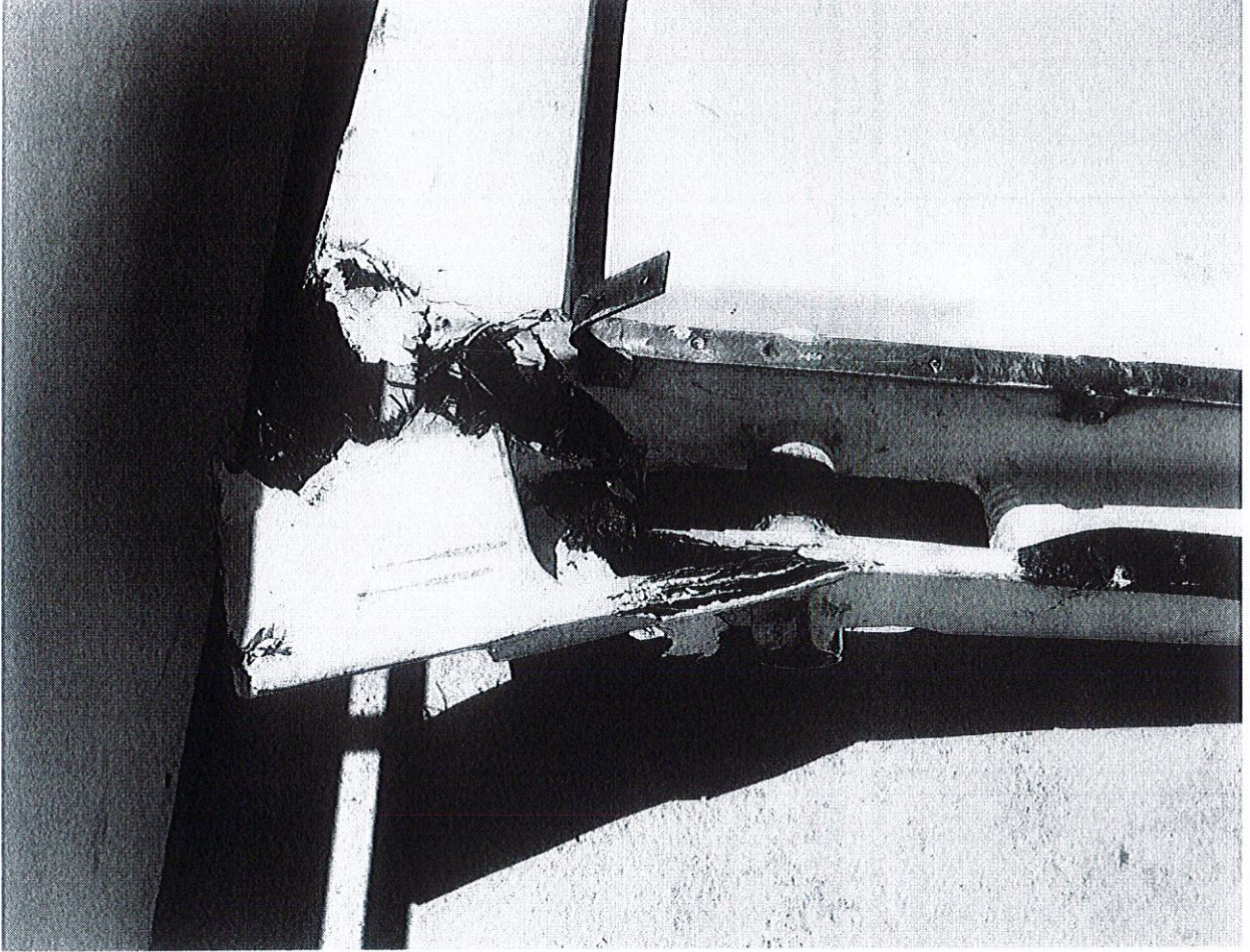
Hasarlı Flap, Kopan Menteşe Nedeniyle Yırılma
