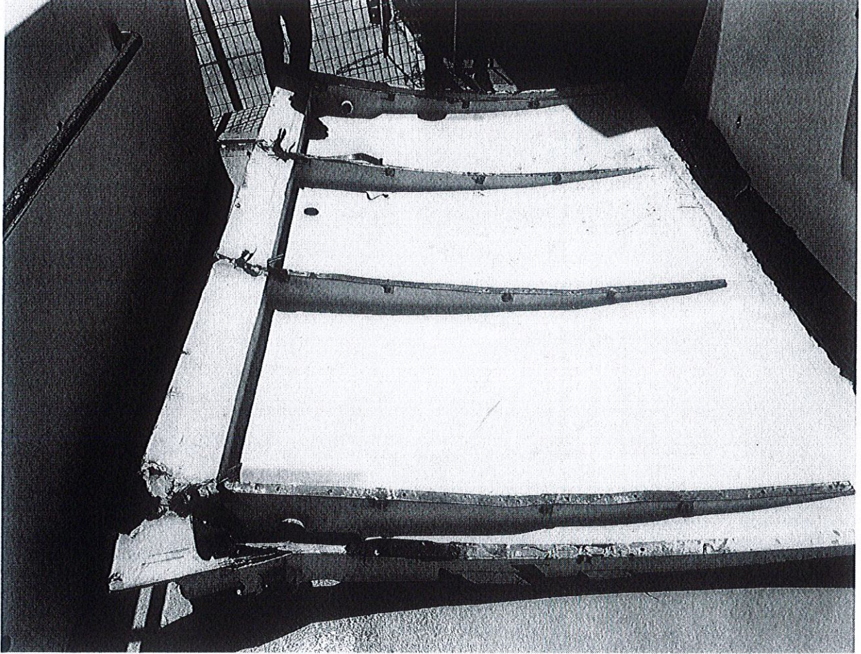
Hasarlı Kompozit Flap
